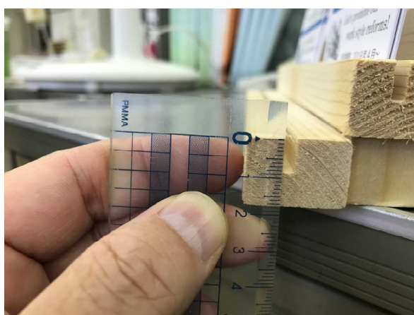
木の厚さは2cm、 溝の深さは8mm くらい
