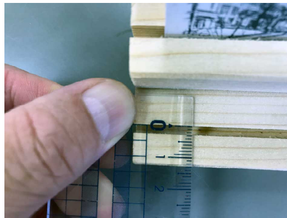
溝の幅はカードが少し倒れてみやすくなるように 幅3mm でつくります
